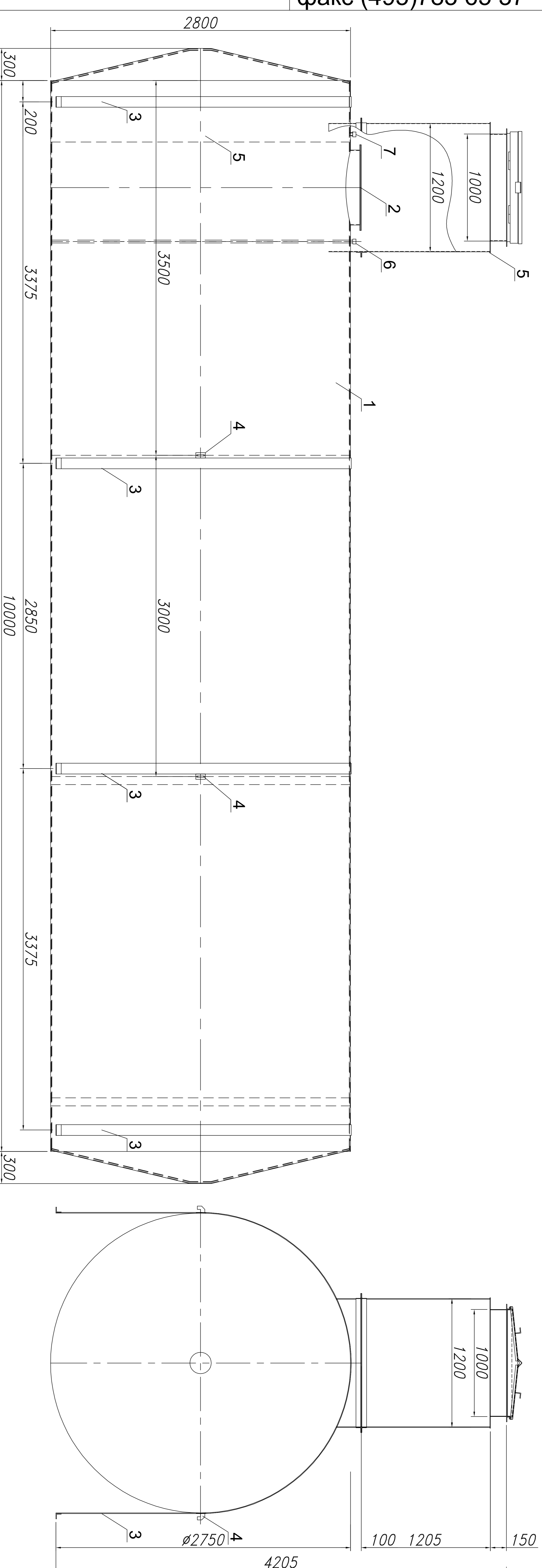
Резервуар РГЦ60
